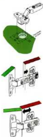
Установка дверей
