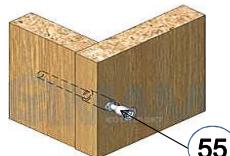
Евровинт 7 x 50
